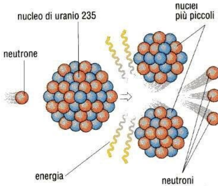
Fissione nucleare
